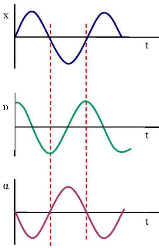
Σχήμα 2. Γραφικές παραστάσεις x = f(t) , v = f(t) και a = f(t) σώματος που εκτελεί γραμμική αρμονική ταλάντωση.
