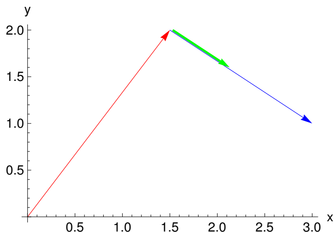
Σχήμα 5.4 - 1: Η Εξίσωση (5.4–2) στο \mathbb{R}^2 όπου \mathbf{r}_A το κόκκινο, \mathbf{n} το πράσινο και \mathbf{a} το μπλε διάνυσμα
