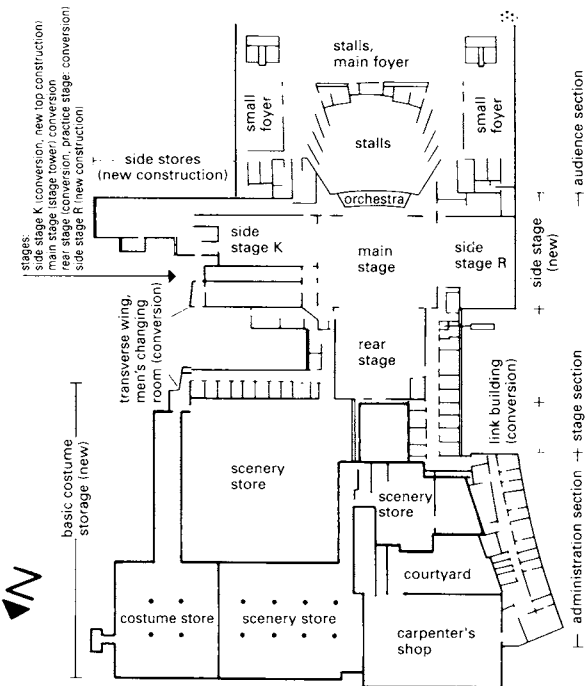
4 Deutsche Oper, Berlin (plan view)
