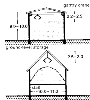
⑤ Hay loft
