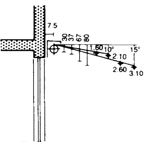
19 Adjustable awning
