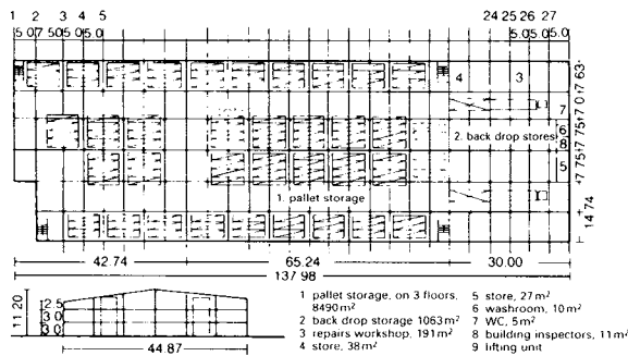
4 Deutsche Oper, Berlin (plan view)
