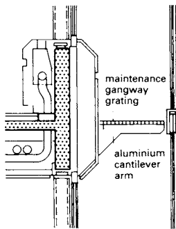
5 Maintenance gangway
