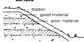
4 Layered fill
