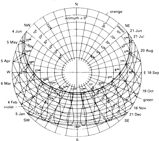
8 Solar position chart for latitude 49°52'N, longitude 8°39', time reference meridian: longitude 15°00'
