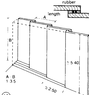
13 Telescopic door
