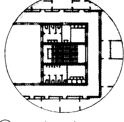
10 a service core in Vereinigten Stahlwerke
