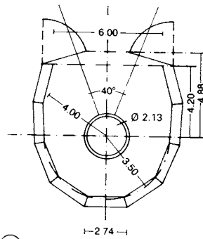
2 Hammer: plan
