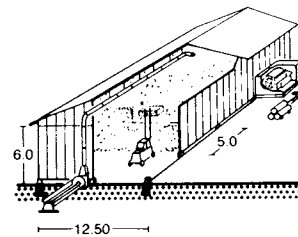
④ Hay storage barn
