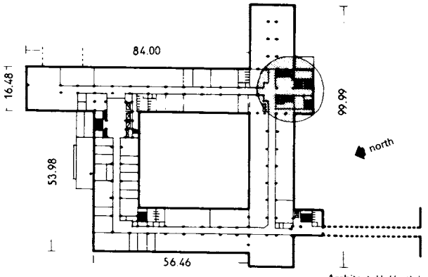
8 Wernerwerke HQ in Siemensstadt, Berlin
