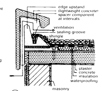
8 Concrete edge profile
